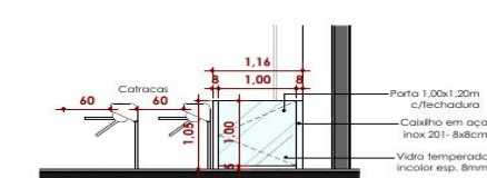
3 DV-02 1 : 50
