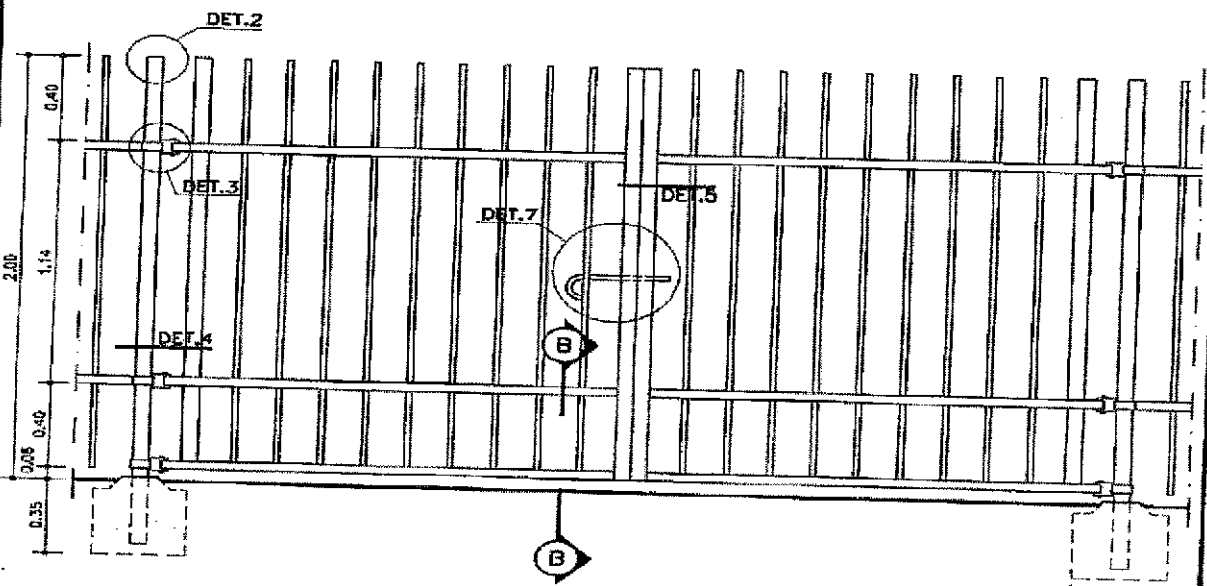
ELEVACAO 1 - PORTAO DE 2 FOLHAS ESC. 1:25
