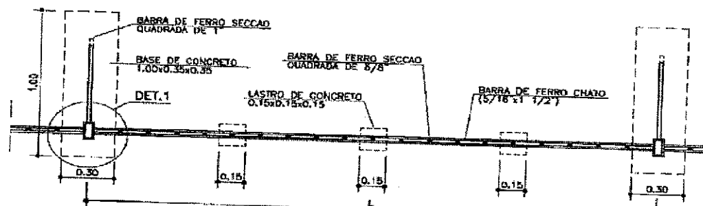
PLANTA ESC. 1:25
