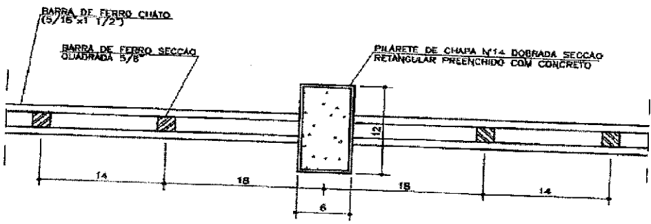
DETALHE 1 ESC. 1:5
